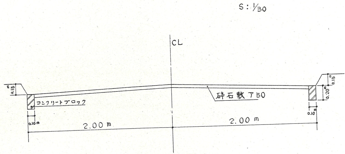
断面図
