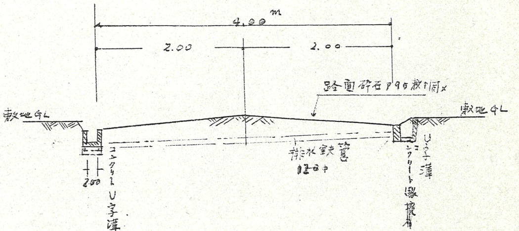
断面図 S 1/50
