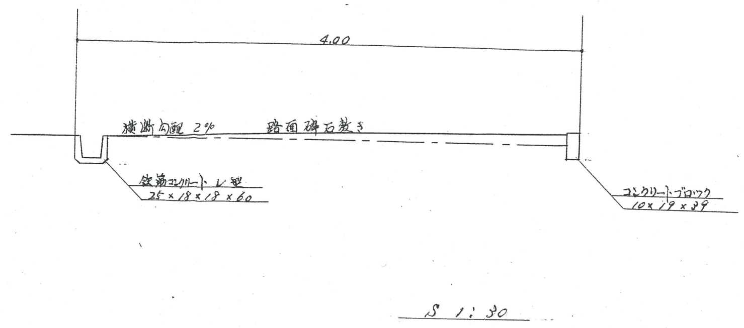
断面図
