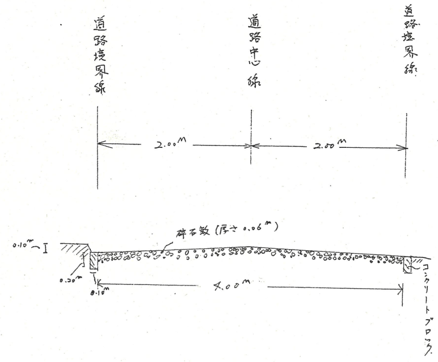
断面図 1/50
