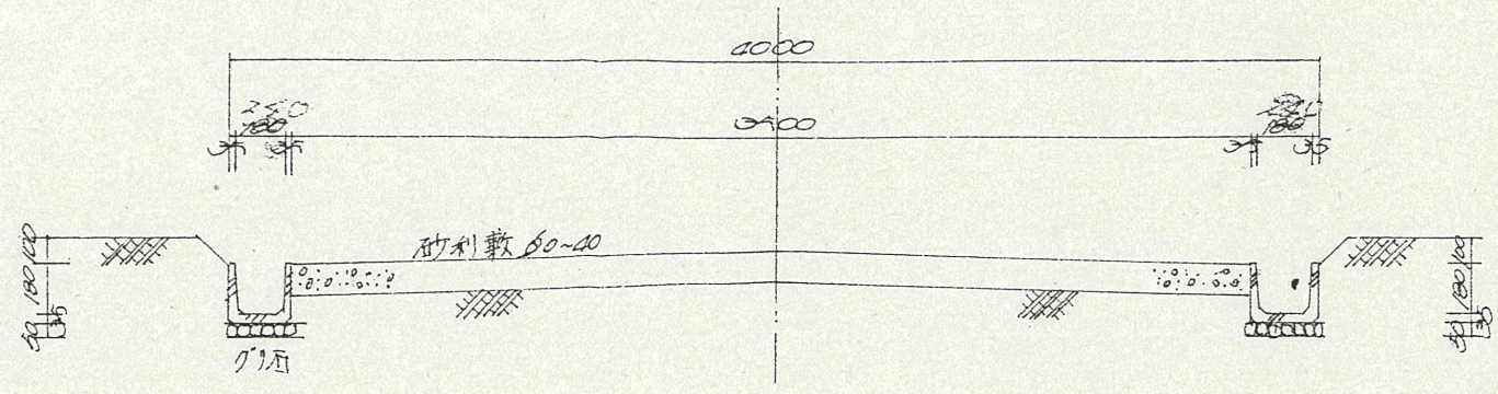
断面図 S=1/30
