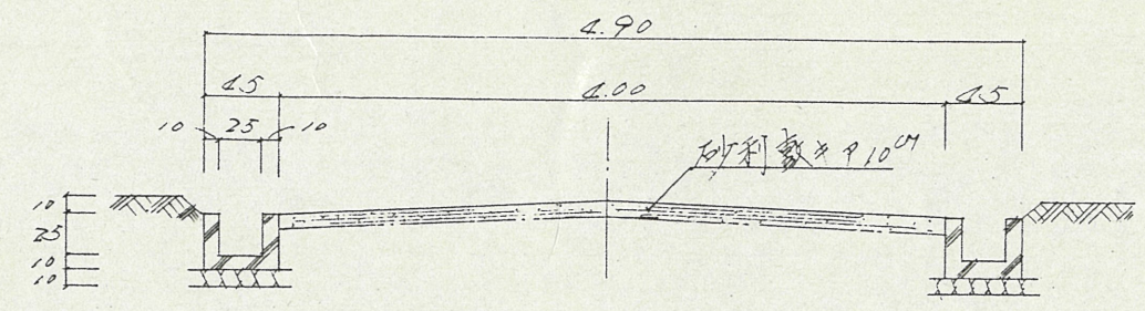
断面図 5. 1/50
