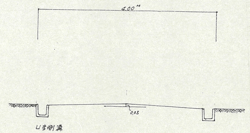
断面図 縮尺 1/50
