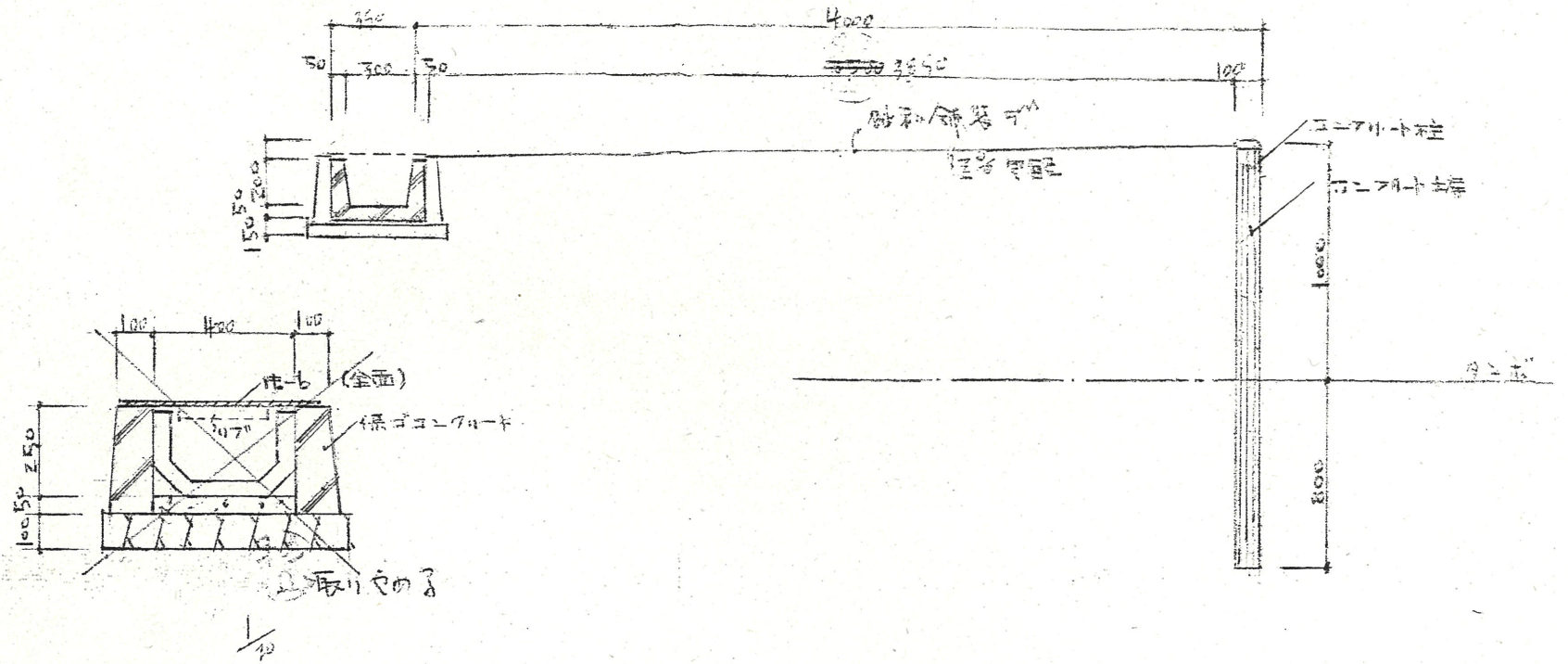
断面図
