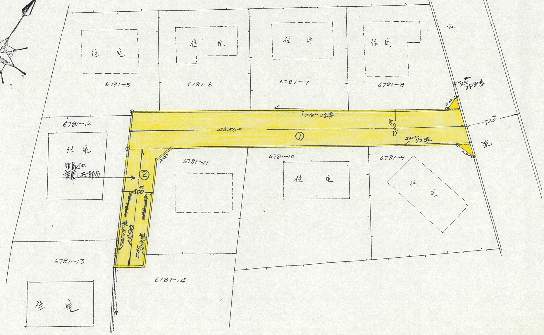
実測図 1/300
