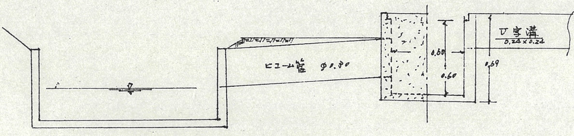
集水軒断面図
