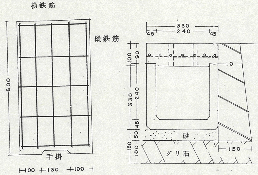
(横断蓋) 縮尺 = \frac{1}{10} (単位: センチメートル)
