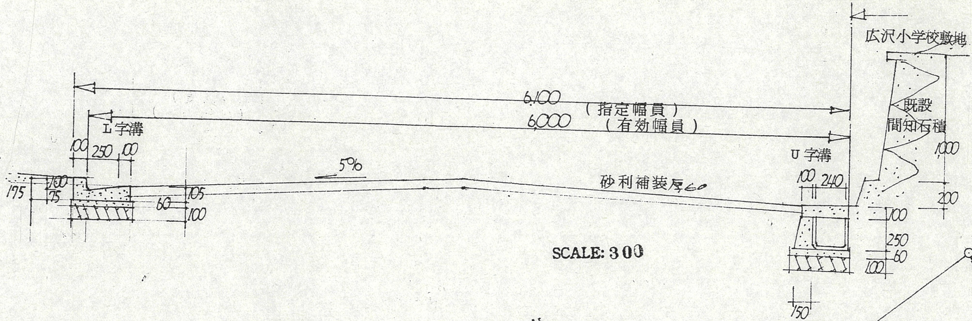
断面図 SCALE: 30
