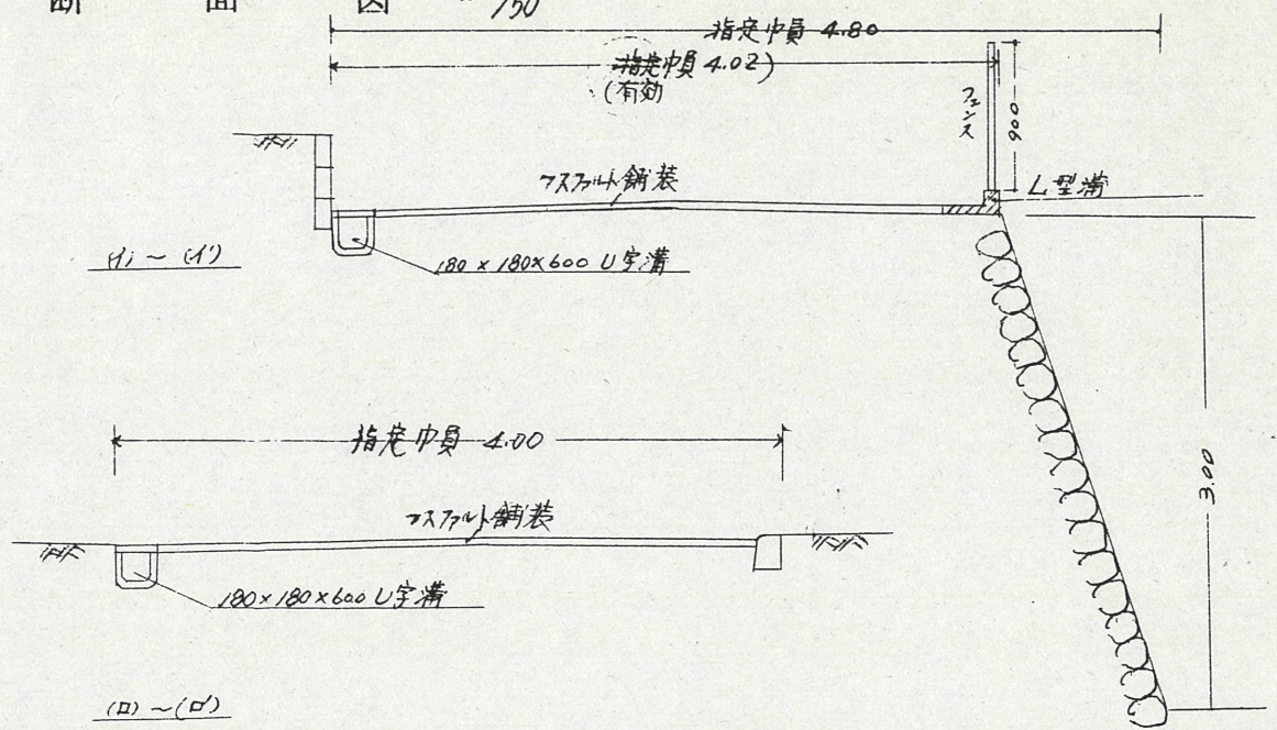
断面図 S-1/50
