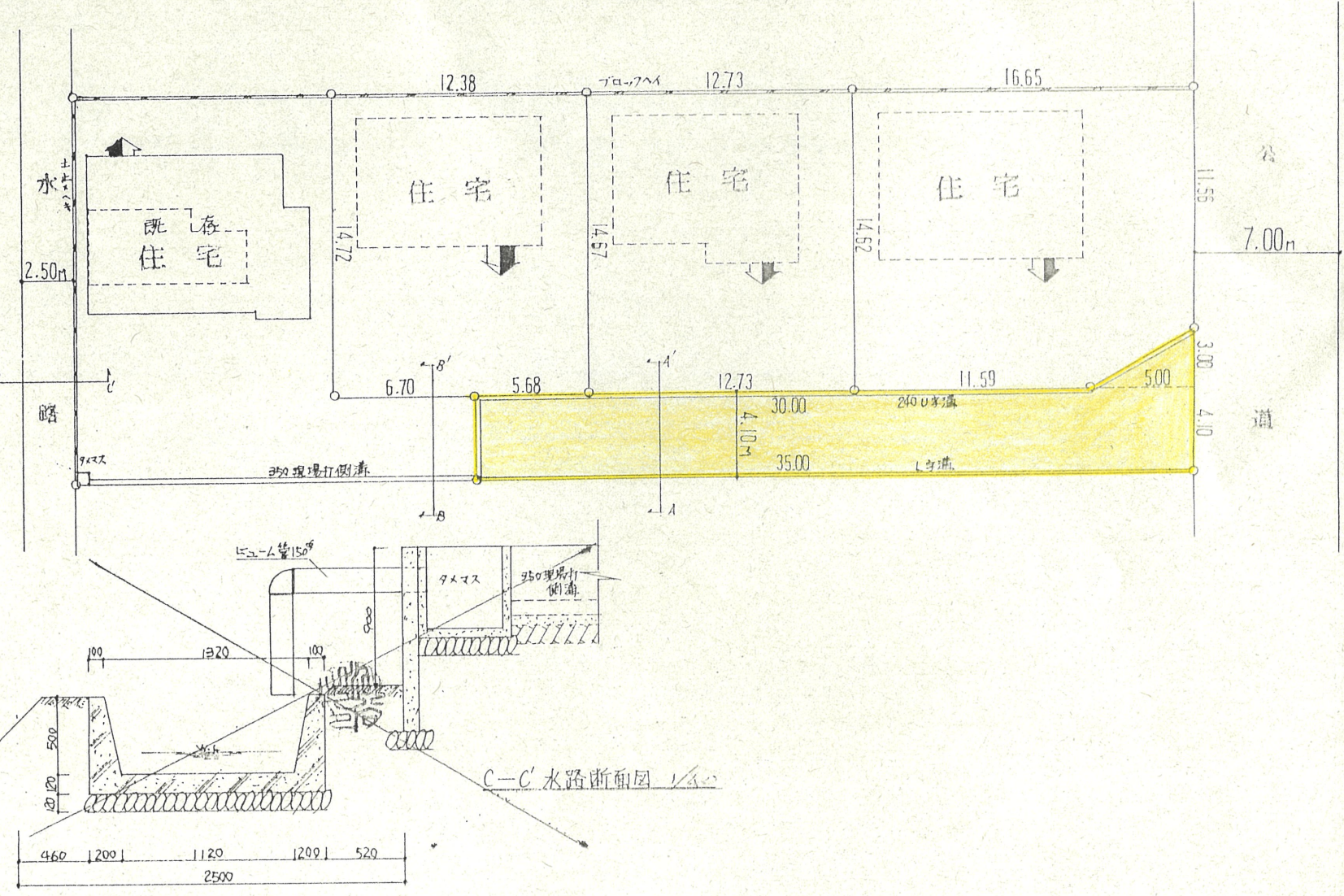
実測図縮尺 1:300
