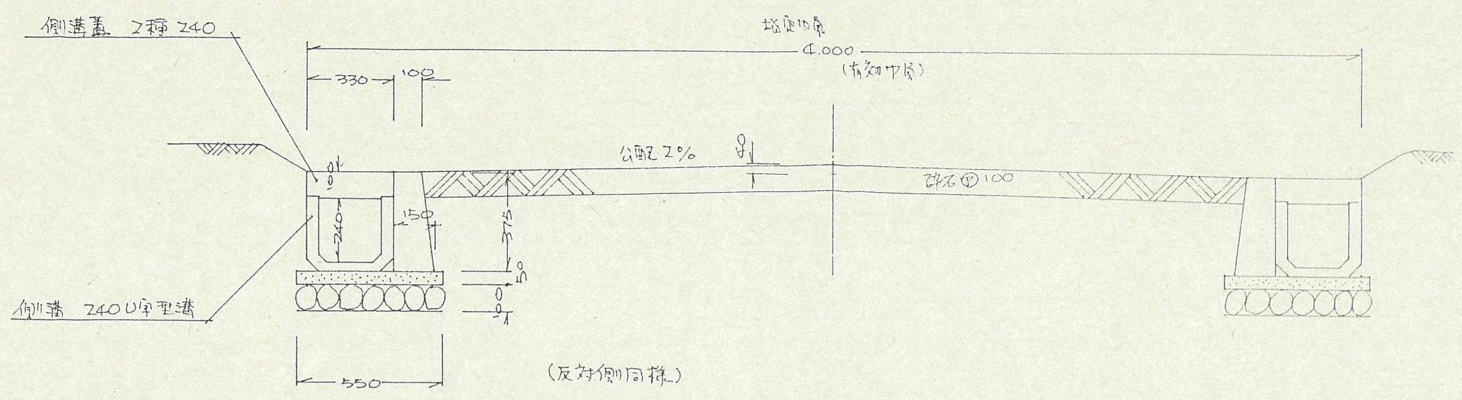
断面図 縮尺 1/20
