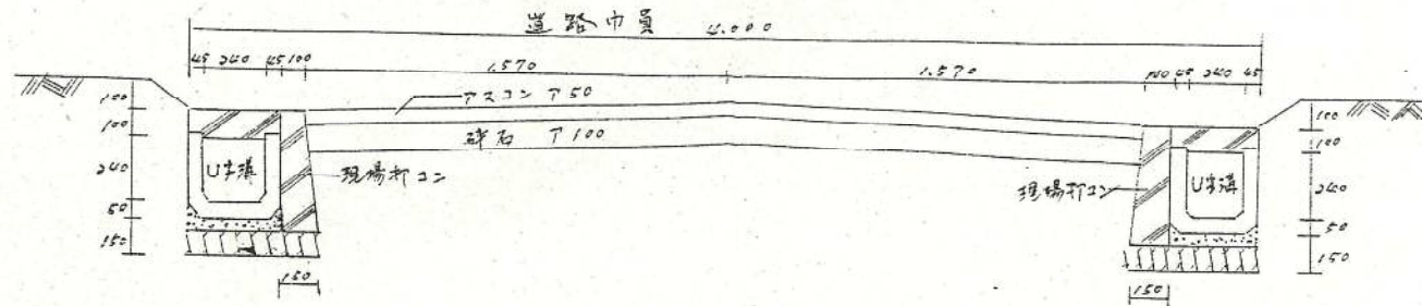
実測図 1/250
