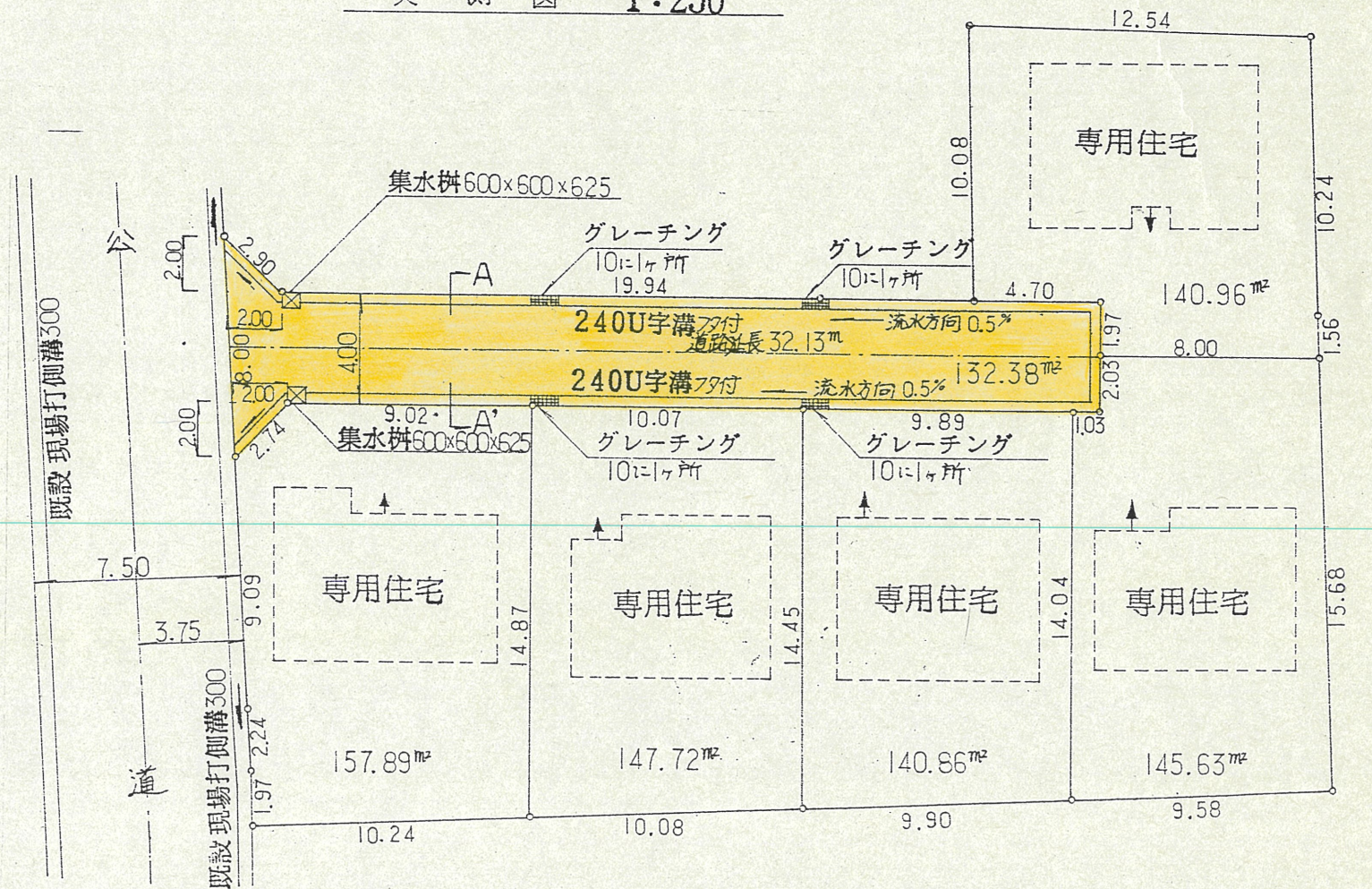
実測図 1:250
