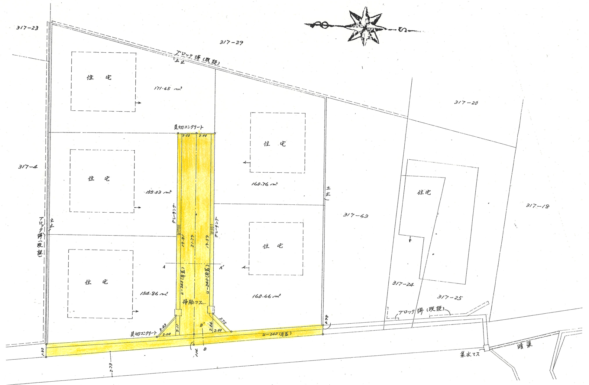
実測平面図
