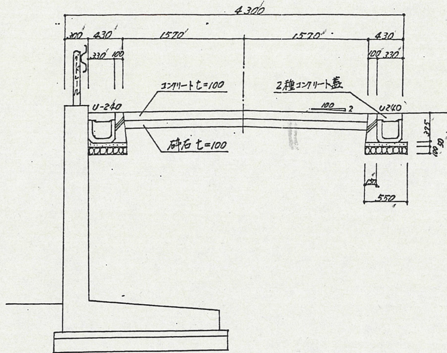
道路断面図 (A-A')
