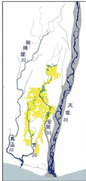
安間川浸水想定区域図
