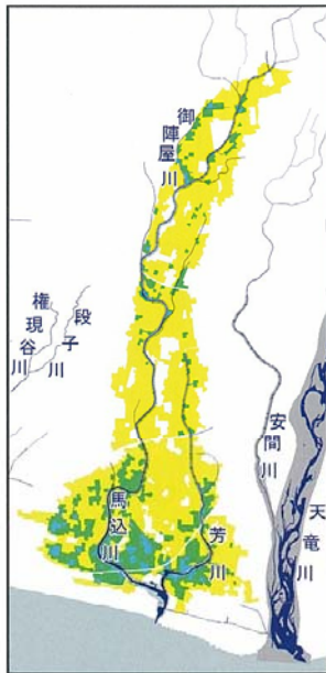
馬込川浸水想定区域図
