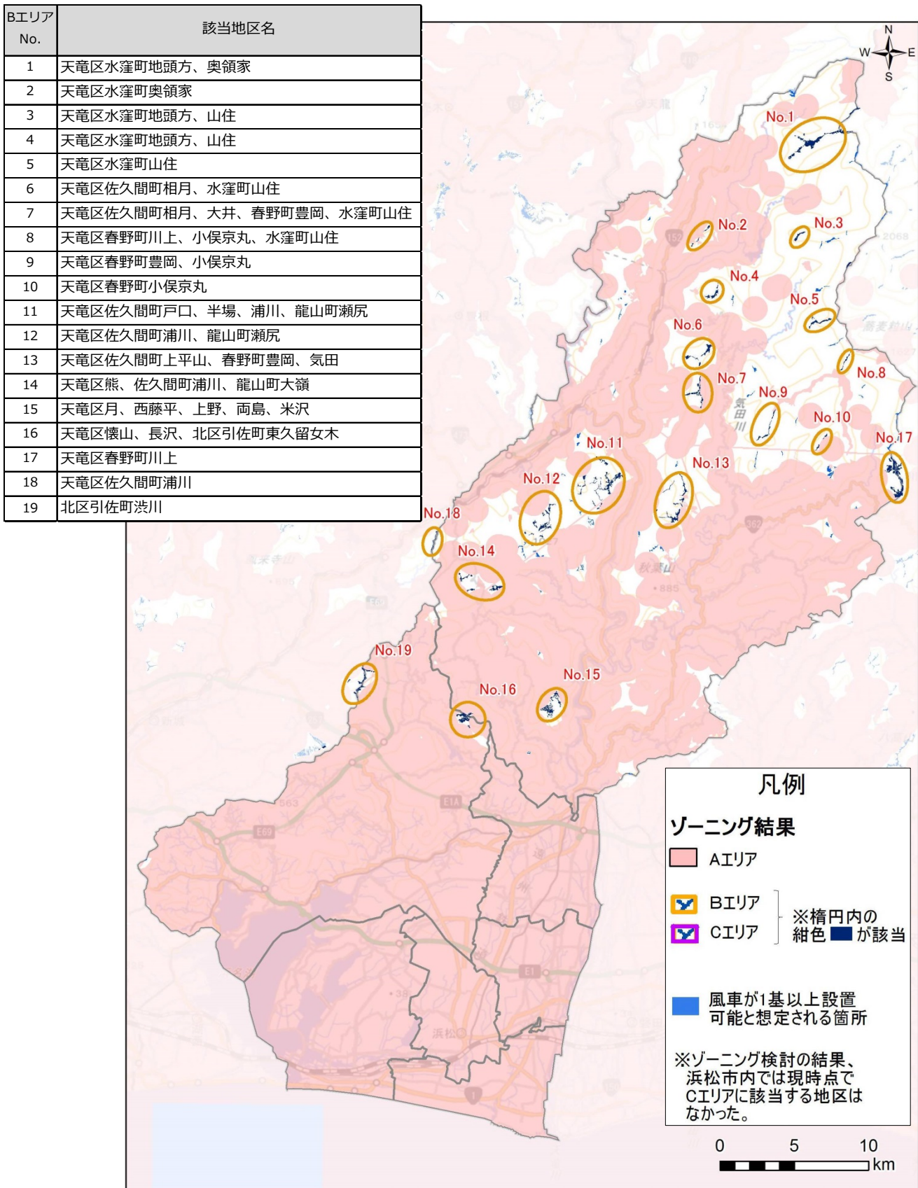
図7 浜松市陸上風力ゾーニングマップ
